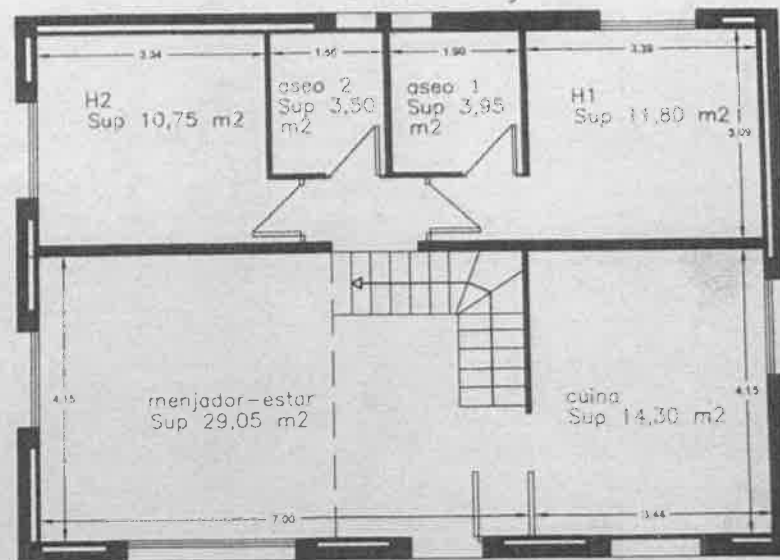
CASA 2-B CASA 4-B Primera Planta
