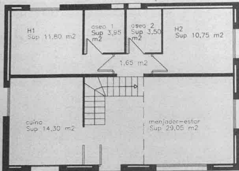
CASA 1-A CASA 3-A Primera Planta
